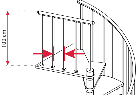
Ø120 Ø140 Ø160 10.8 cm 13.1 cm 15.1 cm
