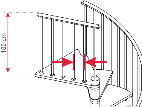
Ø120 Ø140 Ø160 7.0 cm 8.6 cm 10.1 cm
